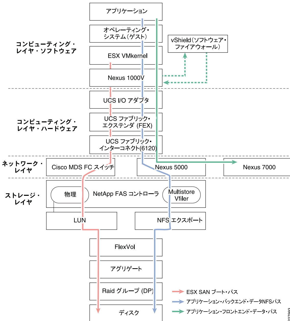
図3 エンドツーエンドのブロック図
