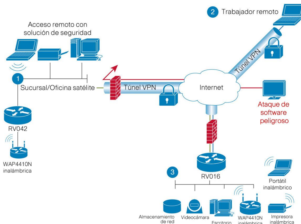
Figura 3. Configuración típica
