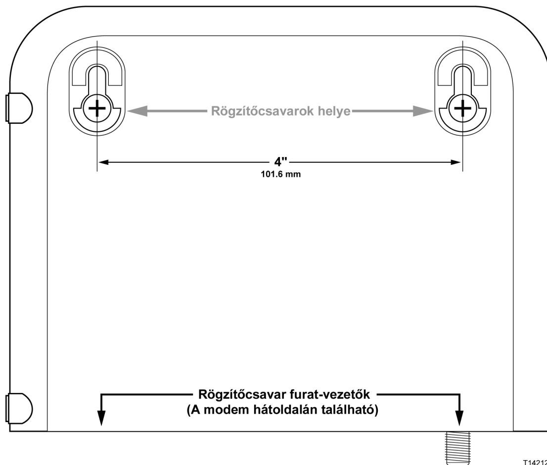
DPC3010 falirögzítés sablonja
