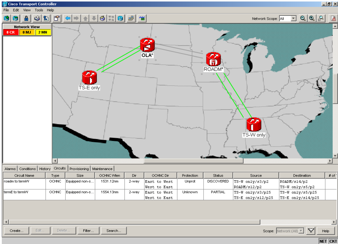
Figure 1-22 Fiber Cut with ALS MODE = Auto Restart
